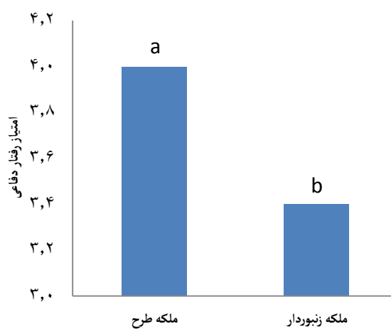
شکل ۴. مقایسه رفتار دفاعی در کلنی‌های اصلاح شده و شاهد
